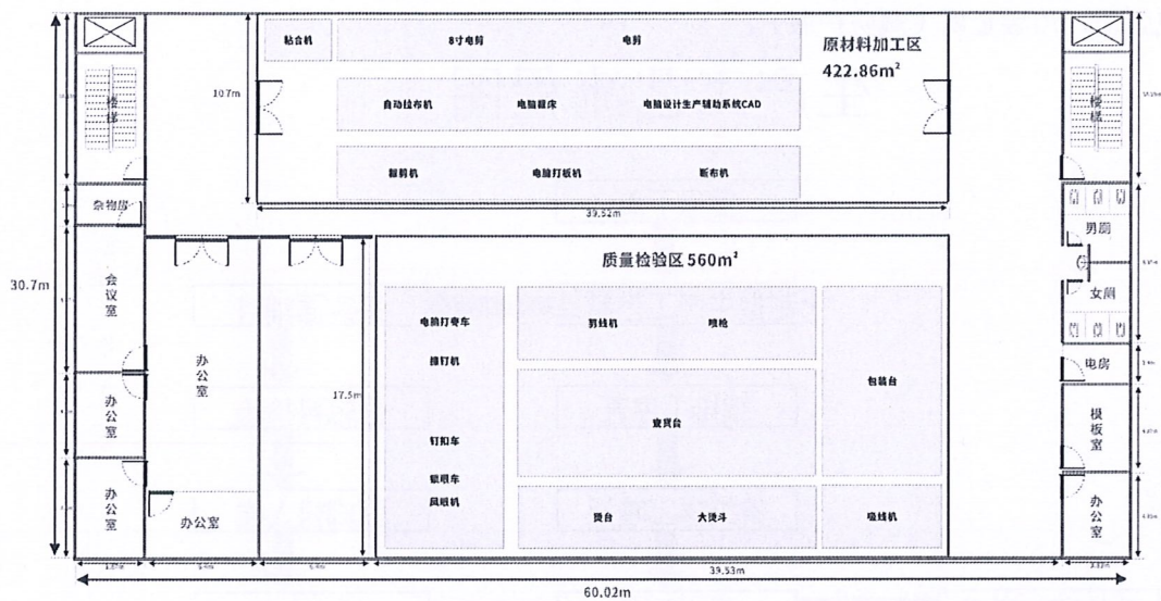
三楼平面图
